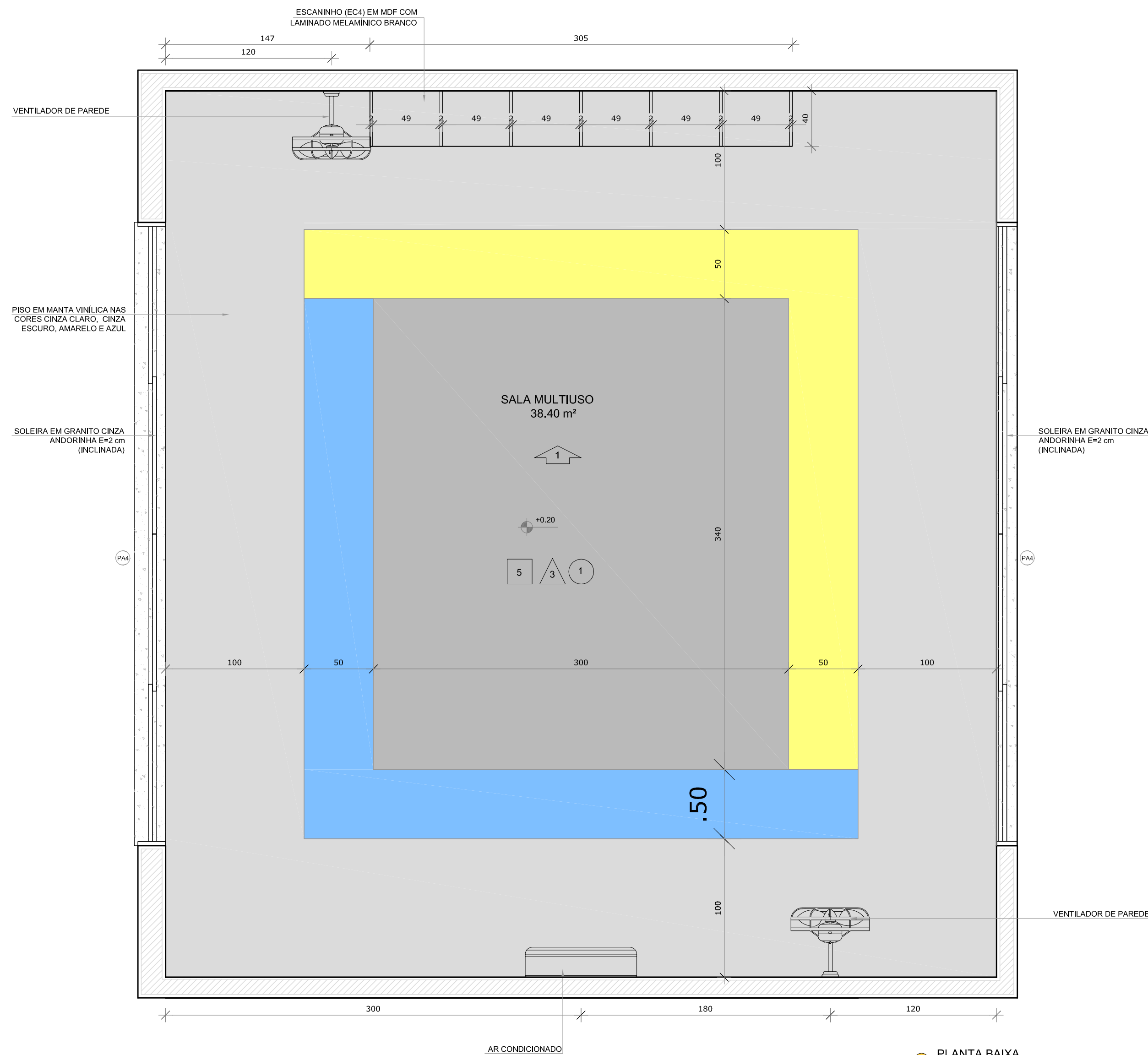
PLANTA BAIXA
